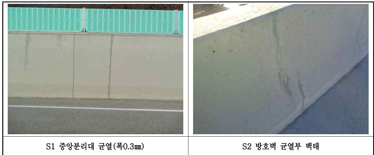
【사진 39.3.21】 방호벽 및 중앙분리대 손상현황
