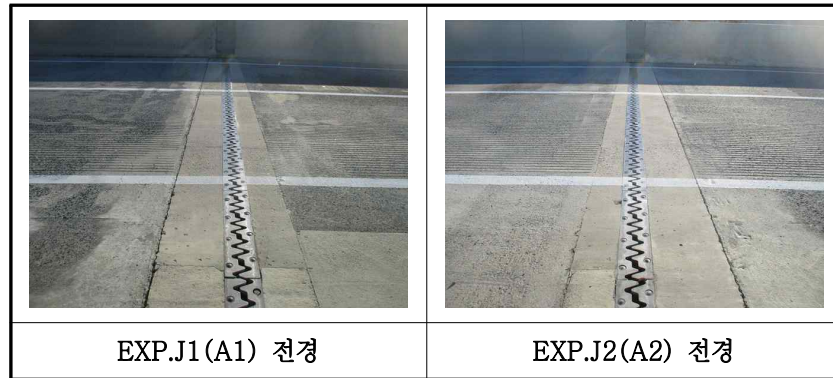
【사진 39.3.32】 신축이음장치 전경
