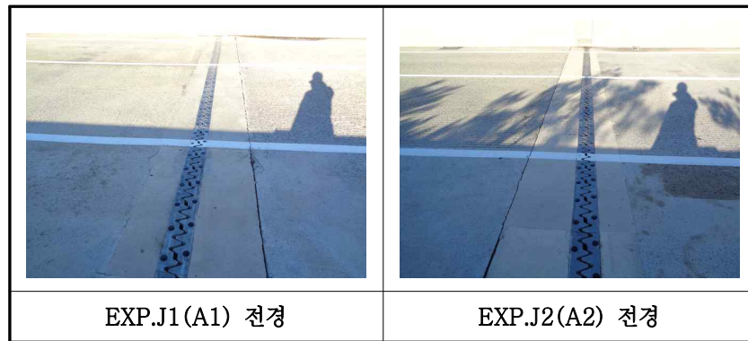
【사진 39.3.14】 신축이음장치 전경
